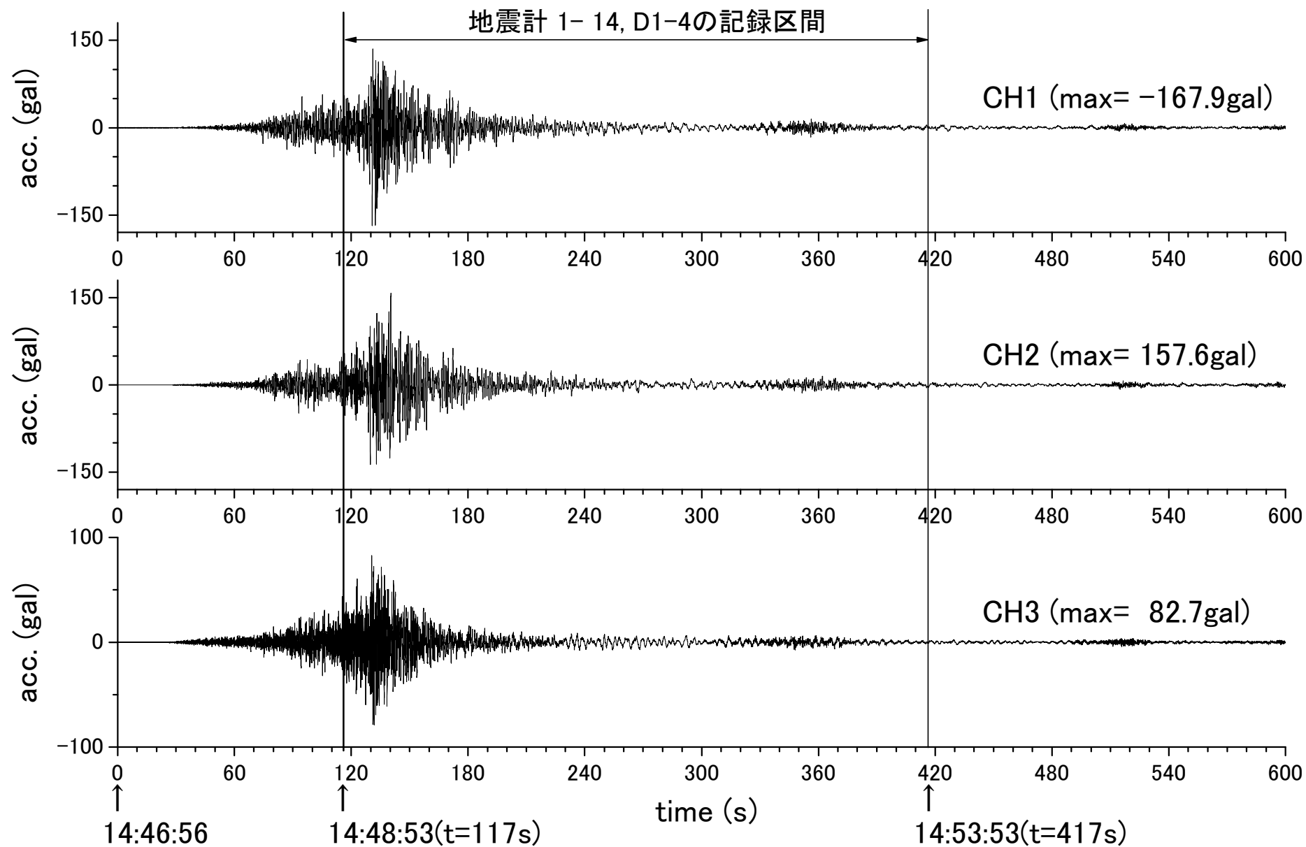
2011年3月11日 東北地方太平洋沖地震(地震計112)
