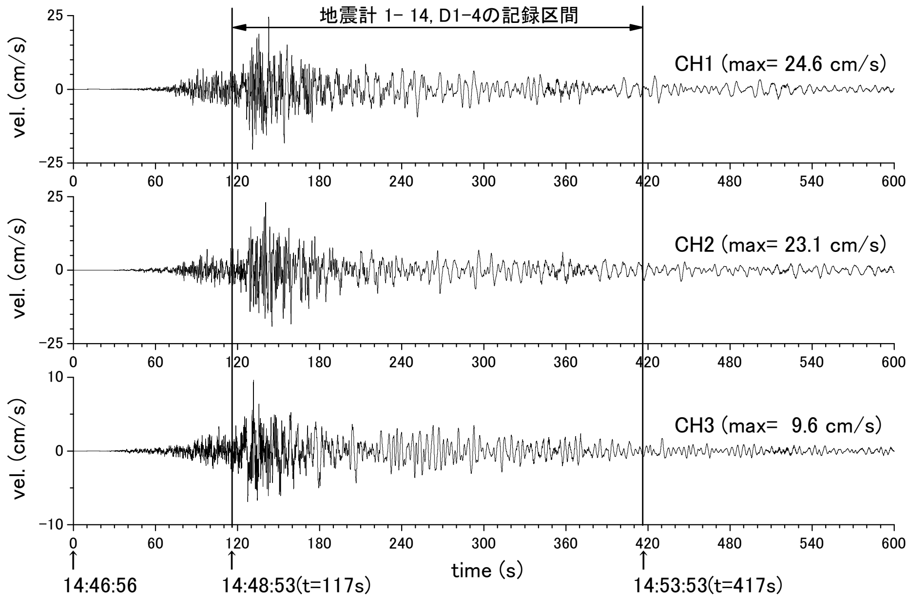
2011年3月11日 東北地方太平洋沖地震(地震計112)
